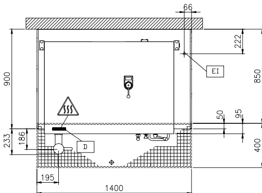
Boven aanzicht
